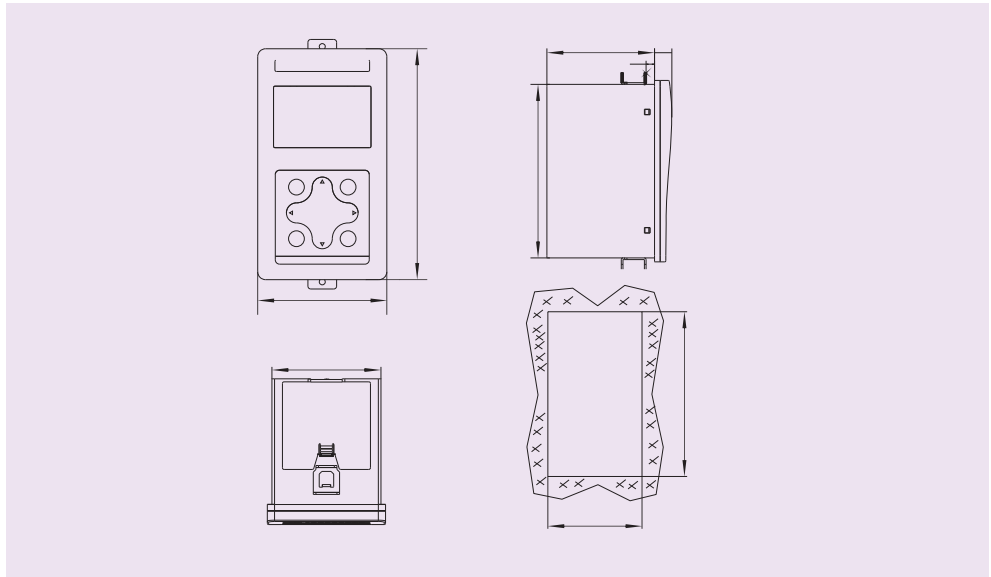
图7 控制器外形及开孔尺寸
