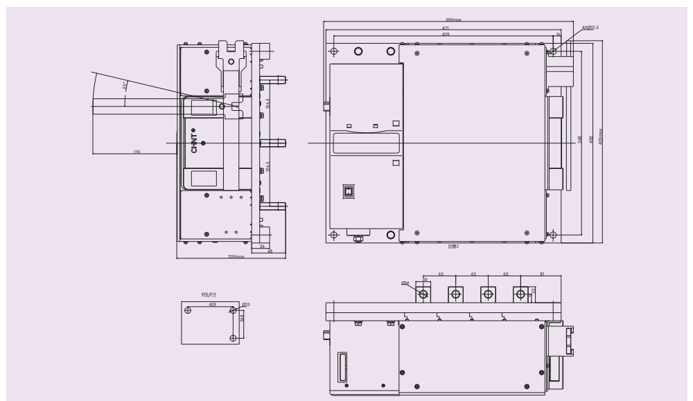
图6 NZ8-800/4 外形及安装尺寸
