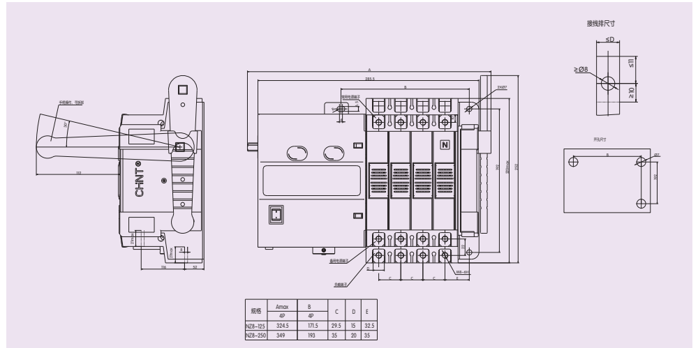
图5 NZ8-400/4 外形及安装尺寸
