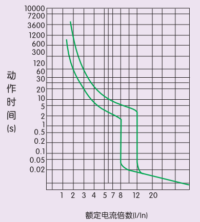
图7 NM7LE-400动作特性曲线
