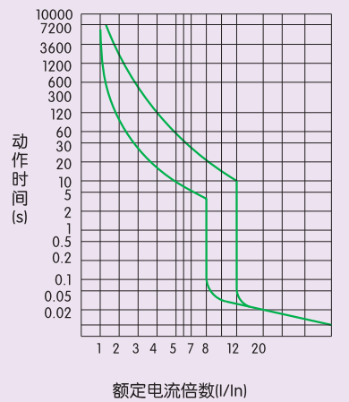
图9 NM7LE-630动作特性曲线
