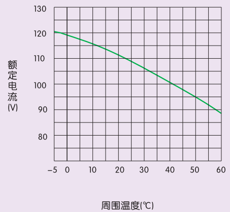
图10 NM7LE-630温度补偿曲线
