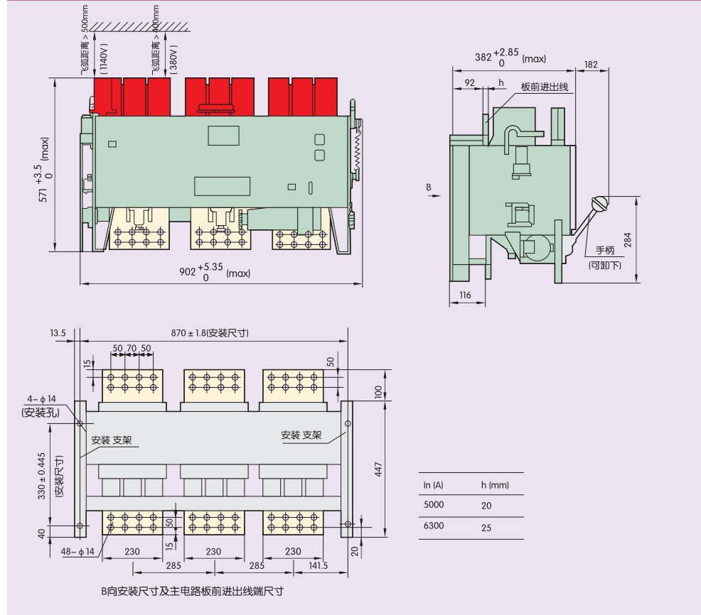
DW15-6300( I_n \geq 5000A )断路器的外形尺寸及安装尺寸
