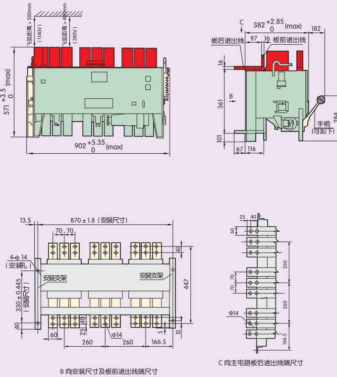
DW15-6300( I_n \leq 4000\text{A} )断路器的外形尺寸及安装尺寸
