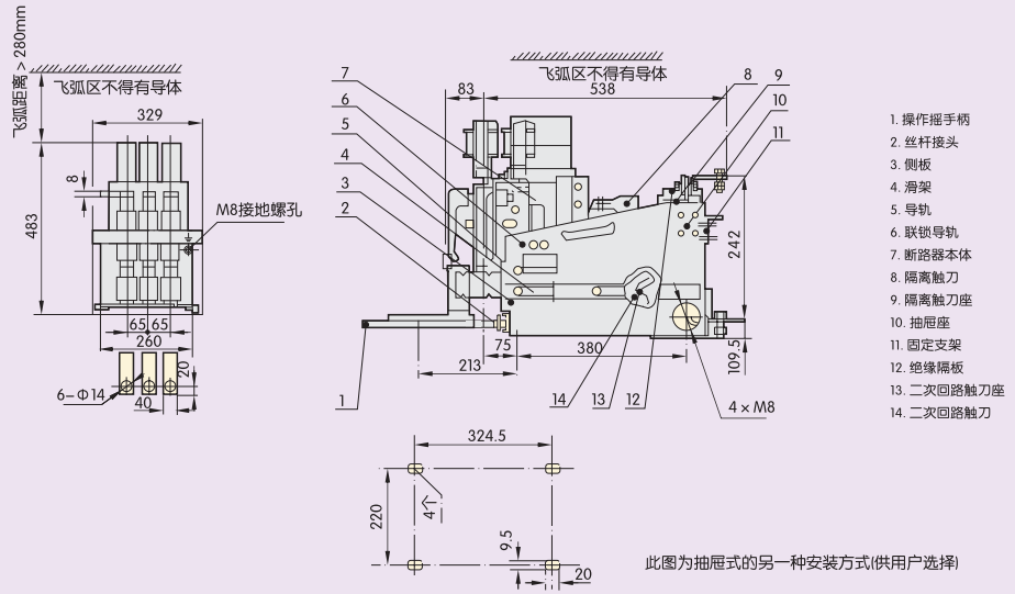
DW15C、DWX15C-630抽屉式断路器外形尺寸及安装尺寸及结构示意图
